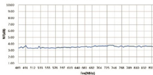
UHF NF
