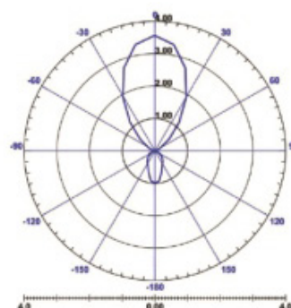
UHF Polar
